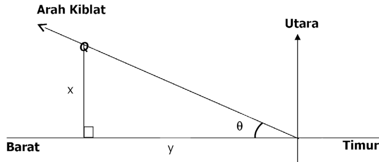
Rajah 5 : Penandaan Sudut Kiblat dari Garisan Timur/Barat
