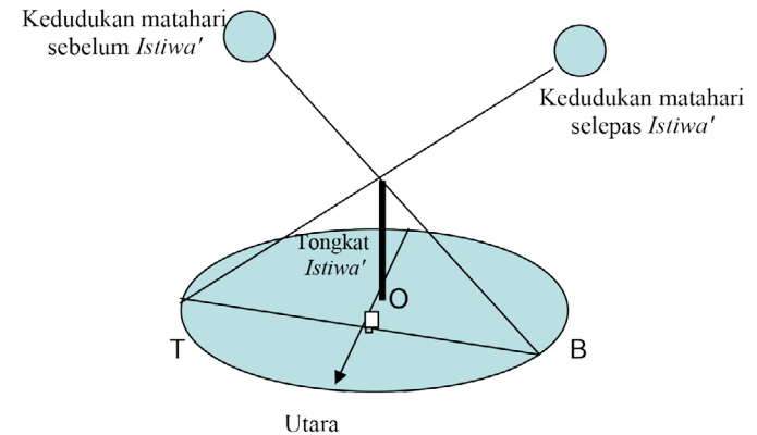
Rajah 4 : Penandaan Arah Utara/Selatan dan Timur/Barat dengan Tongkat Istiwa'
